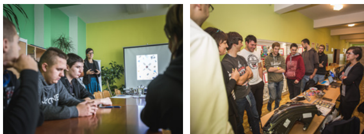
7. 11. 2017 Veletrh firem a pracovních příležitostí
